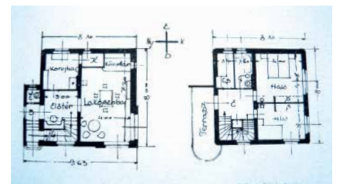
Szende László családi házának alaprajza - Szent L. u. 14. - 1931.
